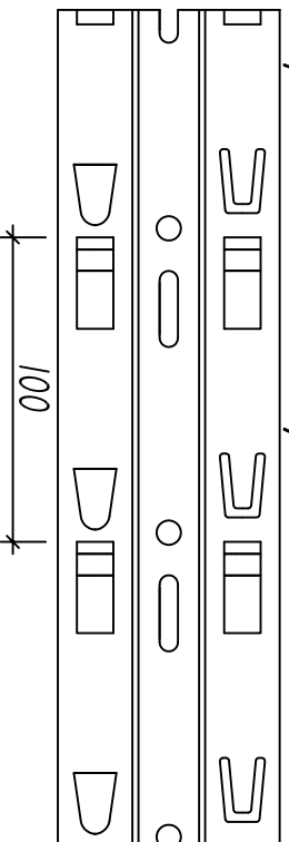
Szynda montażowa TE/100
